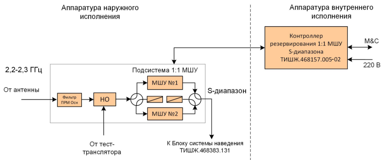
Рисунок 1.1.20 - Структурно-функциональная схема КРМШУ
